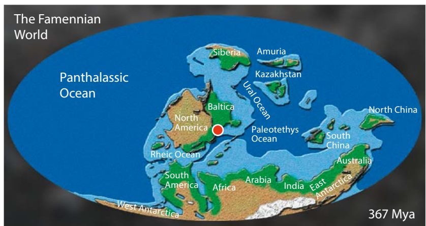
AFBEELDING 9. | Reconstructie van de ligging van de continenten vlak na de overgang van Frasnien naar Famennien in het Boven-Devoon (367 miljoen jaar geleden). De huidige vindplaats Boussu-en-Fagne, Ardennen (oranje ster) lag in die tijd op het continentale plat van vEuramerika/Laurussia (hier aangegeven als North America met Baltica). De vindplaats vormde toen de bodem van een ondiepe zee in de tropische zone ten zuiden van de evenaar. Met dank aan Palaeios en A. White.
